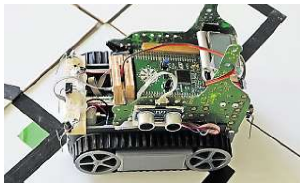
Vier Räder, Leiterplatten und Sensoren gehören zum handtellergroßen Roboter.
